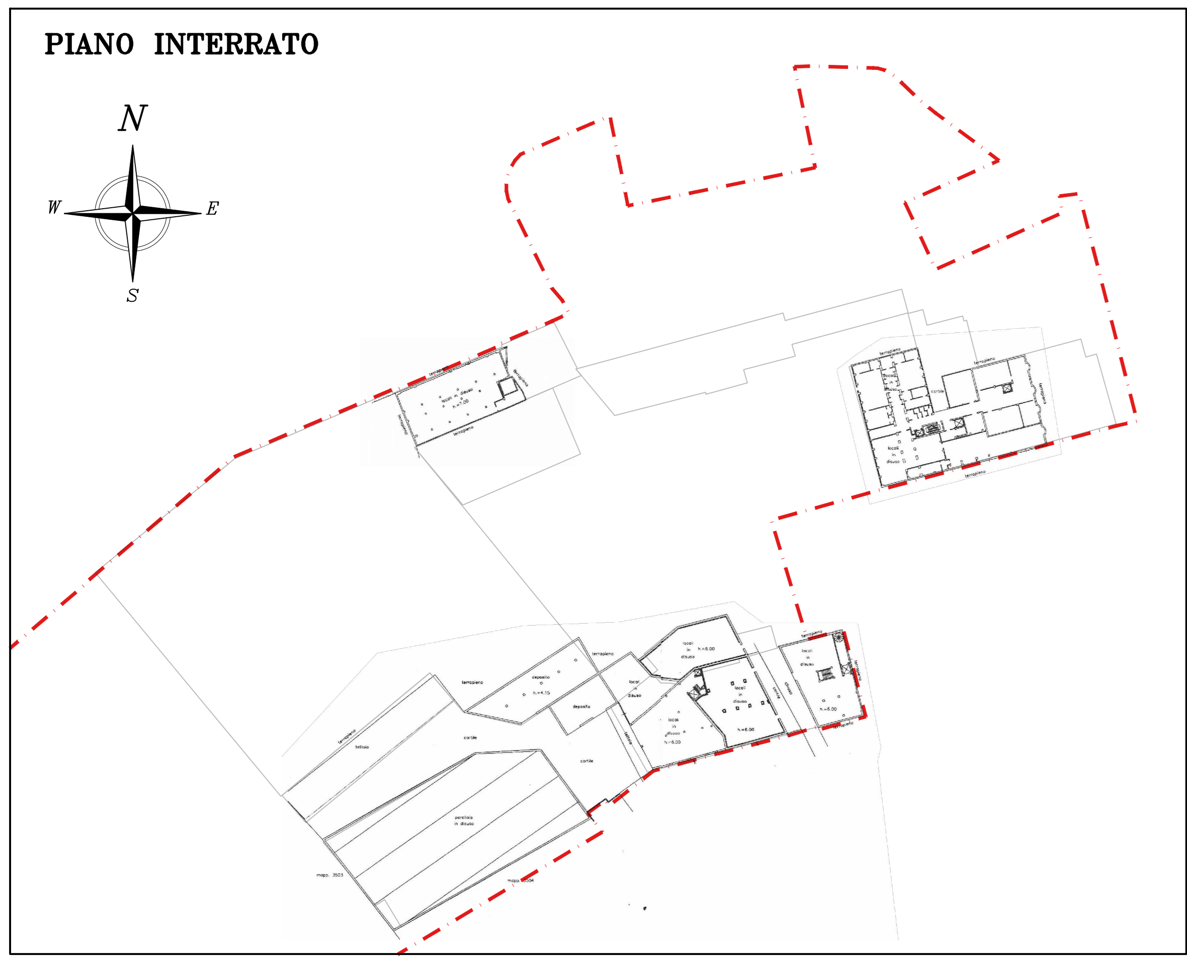
EDIFICI ESISTENTI DA DEMOLIRE scala 1:1000
