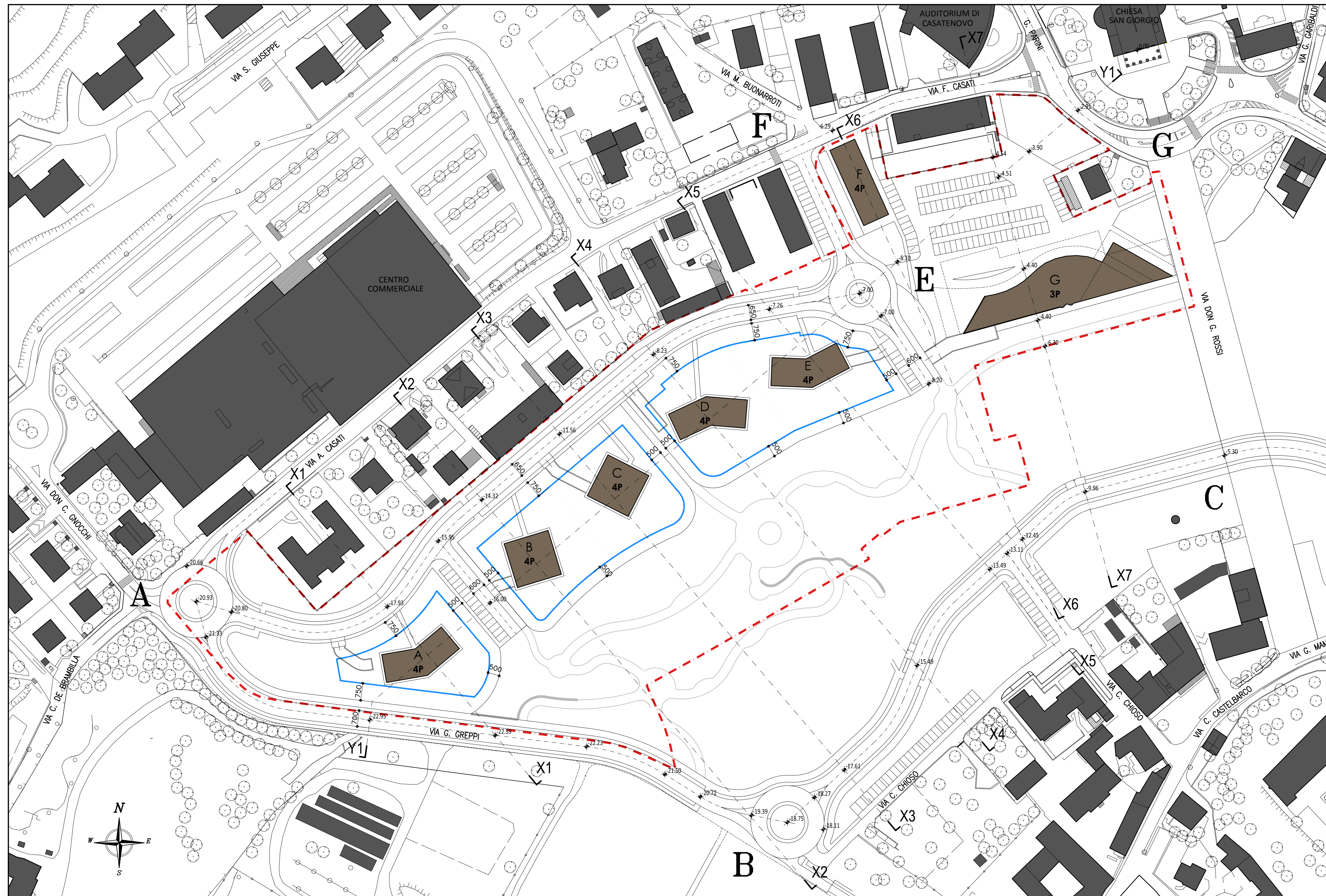
PLANIMETRIA QUOTE ALTIMETRICHE DI PROGETTO-VERIFICA DISTANZE r.1:1000
