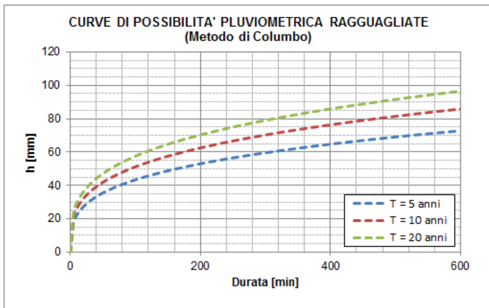
Figura 2 – Curve di possibilità pluviometrica ragguagliate.
