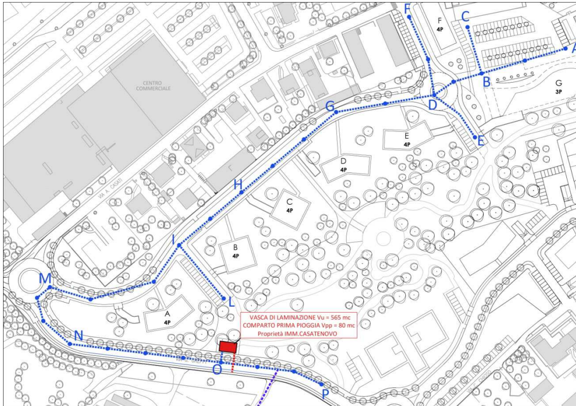
Figura 3 – Schematizzazione rete di smaltimento acque meteoriche Comparto 1.
