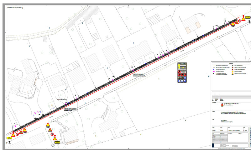
Figura 2 – Layout di cantiere di Via Foscolo.
