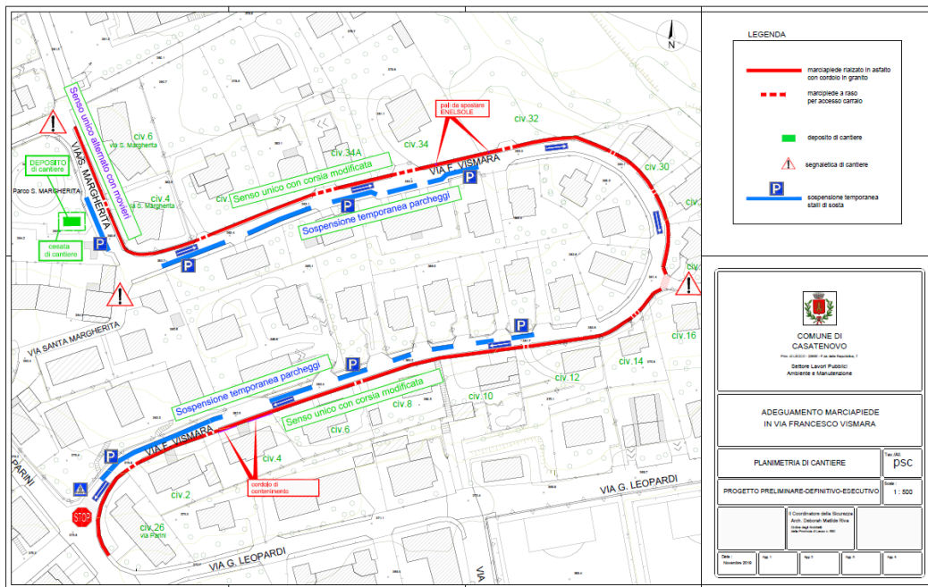
Figura 3 – Layout di cantiere di Via F. Vismara.
