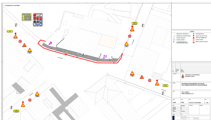
Figura 1 – Layout di cantiere di Via San Gaetano.
